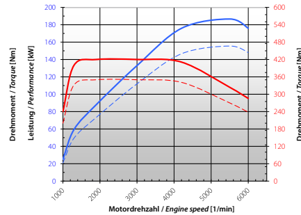
Leistungsdiagramm / Performance chart CB25 Carlsson CB25 vs. 250 CGI (M270)
