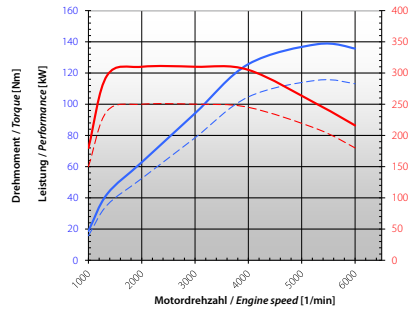
Leistungsdiagramm / Performance chart CB20 Carlsson CB20 vs. 200 CGI (M270)
