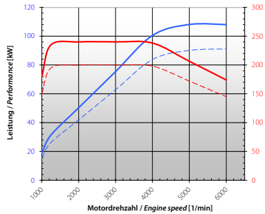
Leistungsdiagramm / Performance chart CB18 Carlsson CB18 vs. 180 CGI (M270)
